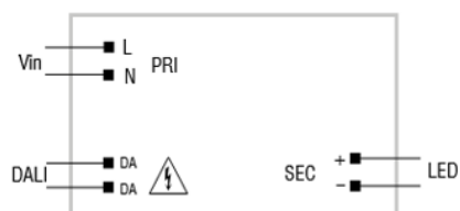
DALI diagram - Collegamento DALI
