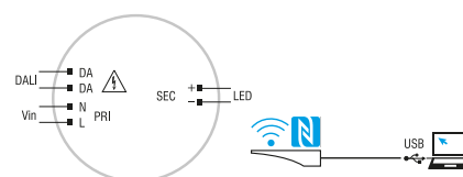
WIRELESS PROGRAMMING diagram Collegamento per PROGRAMMAZIONE WIRELESS
