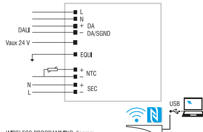
WIRELESS PROGRAMMING diagram Collegamento per PROGRAMMAZIONE WIRELESS
