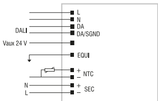
DALI diagram Collegamento DALI
